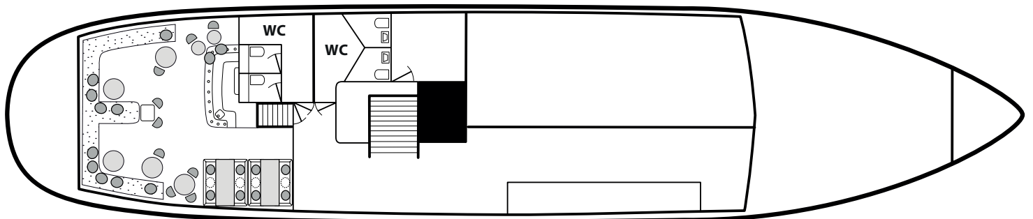
HUVUDDÄCK/MAIN DECK
