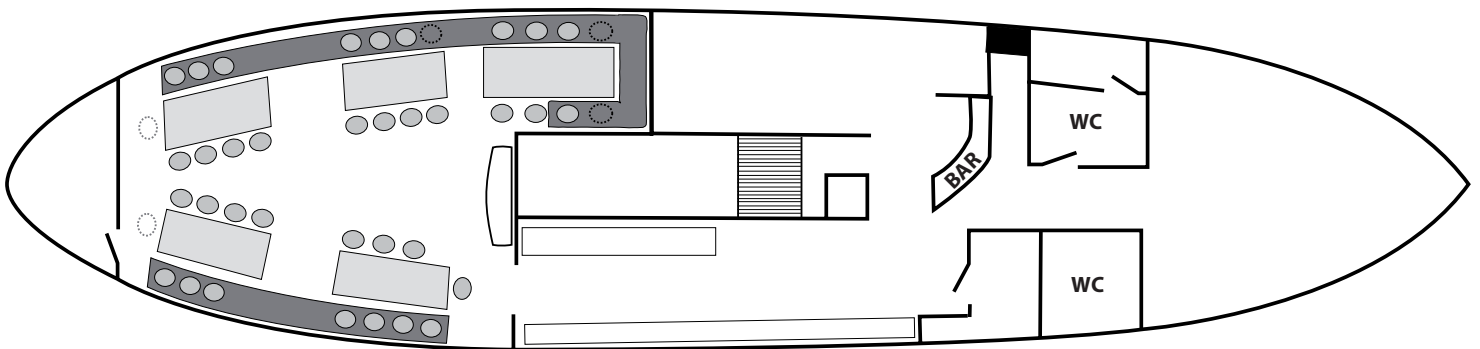
HUVUDDÄCK/MAIN DECK
