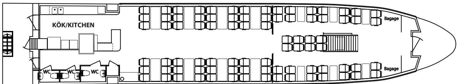
HUVUDDÄCK/MAIN DECK
